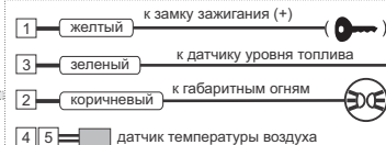
7-контактный разъем переходника
