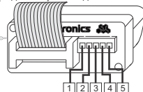
16-контактный разъем OBD-2 (вид со стороны подключения шлейфа)
